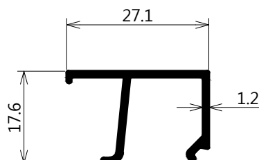
CAS-26721 คิ้วกระทุ้ง 8 มม. WT : 0.200 Kg./M 6 เส้น/มัด
