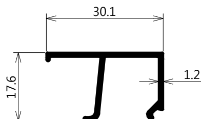
CAS-26396 คิ้วกระทุ้ง 6 มม. WT : 0.209 Kg./M 6 เส้น/มัด
