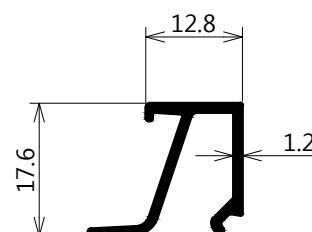
CAS-34010 คิ้วกรอบบาน 30 มม. WT : 0.175 Kg./M (6 เส้น/มัด)
