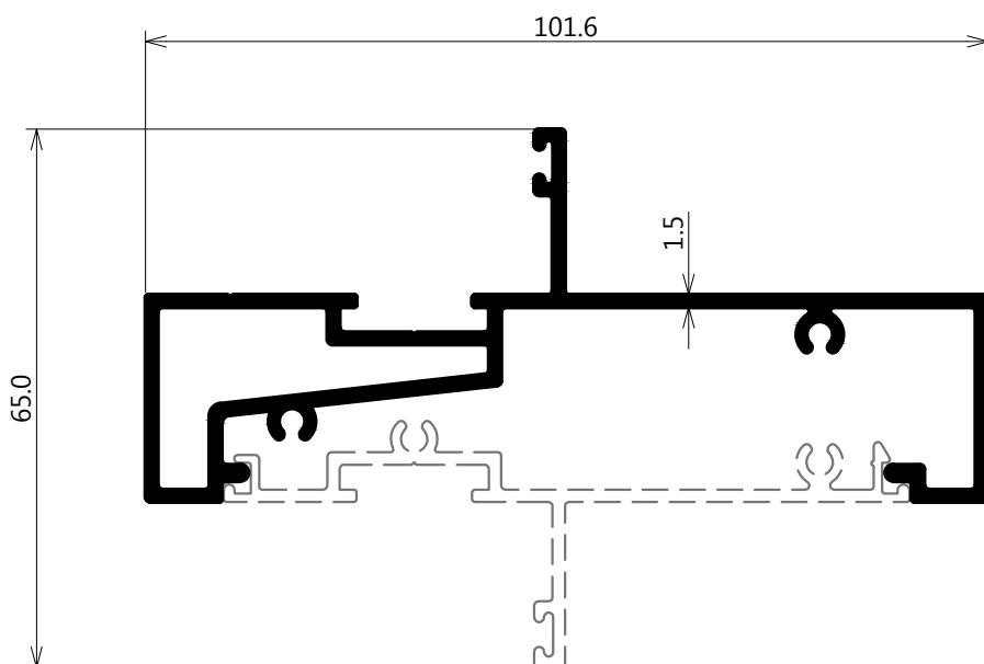
CAS-26568 กรอบนอกบานกระทุ้ง 4 นิ้ว WT : 1.129 Kg./M 2 เส้น/มัด
