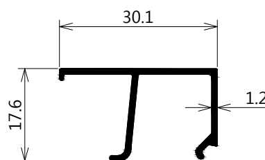
FOL-26396 ก๊วกระทุ้ง 6 มม. WT : 0.209 Kg./M 6 เส้น/มัด
