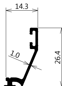
FOL-26499 บังใบบานพับ WT : 0.151 Kg./M 4 เส้น/มัด
