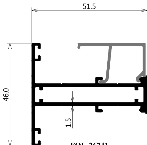
FOL-26741 ชอยกลางบานพับ WT : 0.753 Kg./M 4 เส้น/มัด
