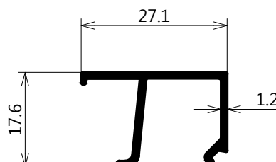
FOL-26721 ก๊วกระทุ้ง 8 มม. WT : 0.200 Kg./M (6 เส้น/มัด)
