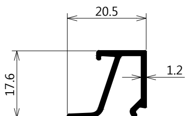
FOL-34010 ก๊วเสาบานพับ 30 มม. WT : 0.175 Kg./M (6 เส้น/มัด)
