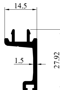
FOL-33245 ดบเสาต่างบานเฟี้ยม WT : 0.232 Kg/M (4 เส้น/มัด)
