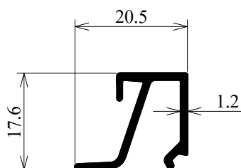
FOL-34010 คิวเสาบานเฟี้ยม 30 มม. WT : 0.175 Kg/M (6 เส้น/มัด)
