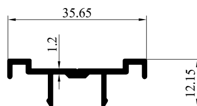
FOL-33241 ดบเฟรมข้าง WT : 0.211 Kg/M (4 เส้น/มัด)
