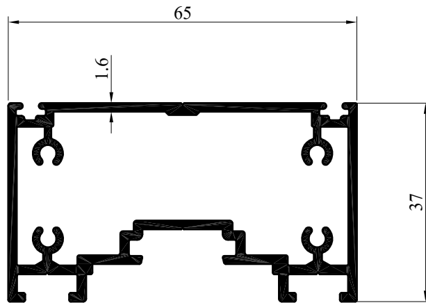
FOL-33242 เสริมเสาบานเฟี้ยมล้อ WT : 1.260 Kg./M (2 เส้น/มัด)
