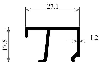
FOL-26721 คิวเสาบานเฟี้ยม 15.70 มม. WT : 0.200 Kg/M (6 เส้น/มัด)
