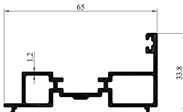
FOL-33244 เสริมเสาบานเฟี้ยมคี่ WT : 0.710 Kg/M (2 เส้น/มัด)
