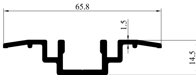
FOL-33243 เฟรมล่างบานเฟี้ยมฝัฟ้น WT : 1.530Kg./M (2 เส้น/มัด)
