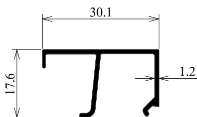
FOL-26396 คิวเสาบานเฟี้ยม 12.70 มม. WT : 0.209 Kg/M (6 เส้น/มัด)
